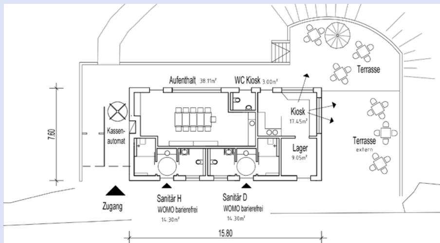
Grundriss Funktionsgebäude Variante III
